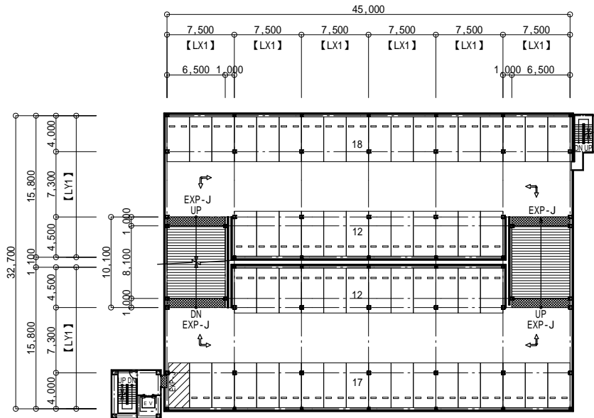
2 ~ 4階 平面図
