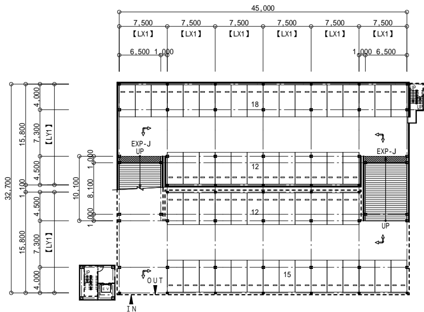
1階 平面図
